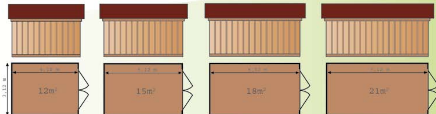
Modèle présenté 3.12 / 5.12 m avec option chassis - réf. GA0251
