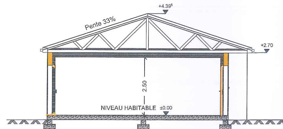
COUPE AA
