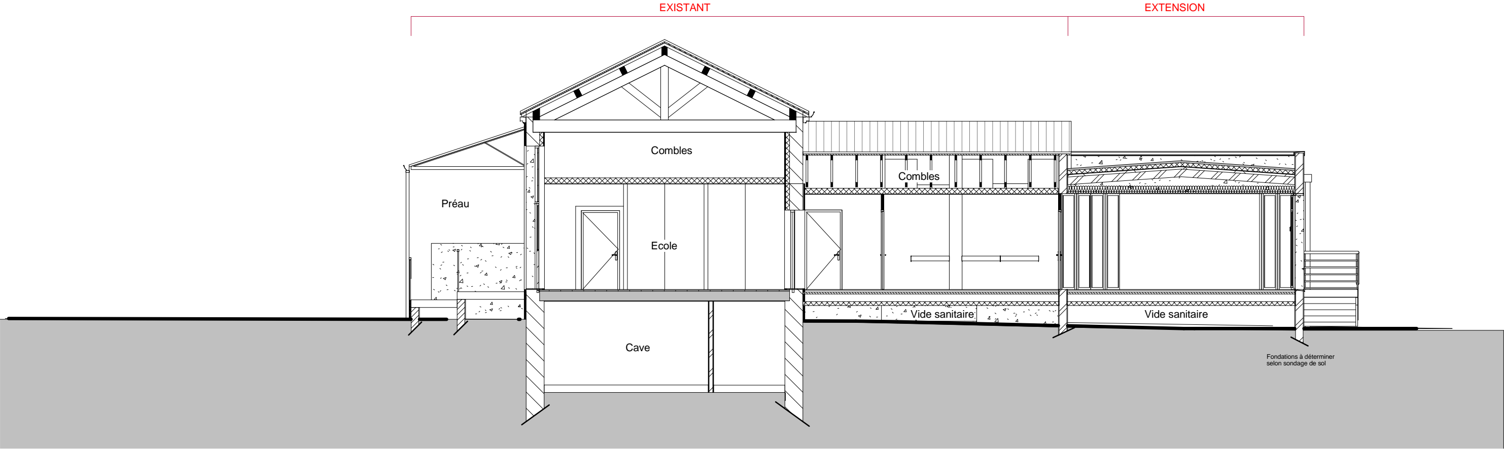
Ecole-Coupe transversale 1 : 100
