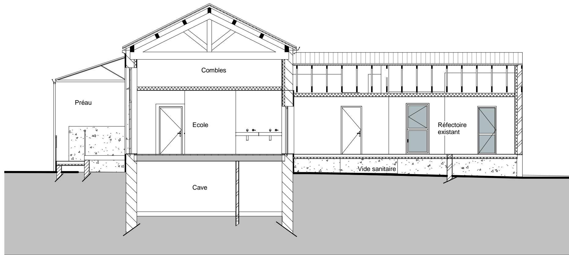
Coupe transversale existante 1 : 100
