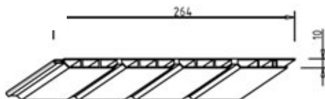
Figure 3 – Lambris de sous face
