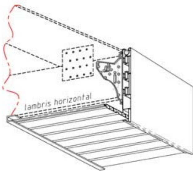
Figure 8a – Avant-toit pose horizontale
