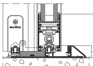
Schüco ASS 41 SC Seuil EasyAccess PMR
