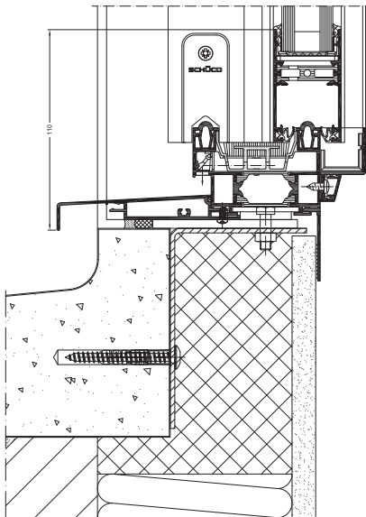
Schüco ASS 41 SC Seuil pose ITI
