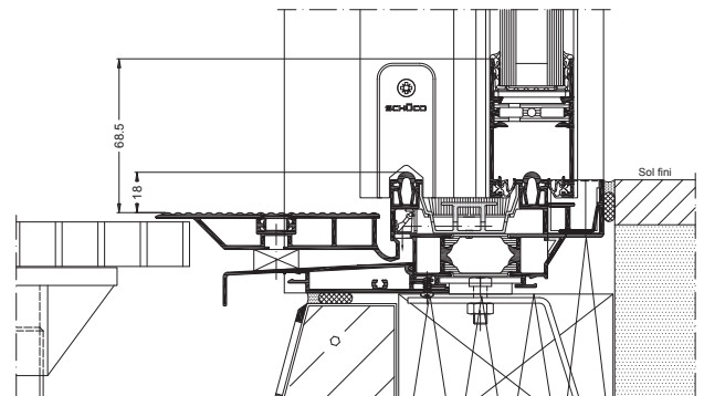
Schüco ASS 41 SC Seuil encastré avec liaison terrasse extérieure (PMR)
